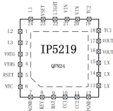
图 2 IP5219 引脚图
